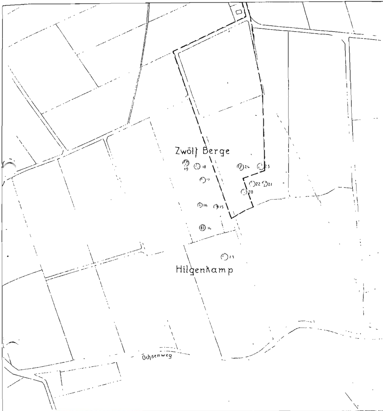
Abb. 324. Oldendorf, Vermessungsplan der Grabhügel 13—24 (1 : 5000).
